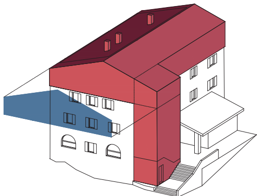
PROGETTO: L'inserimento del corpo scala permette la creazione in facciata di una falda simmetrica
