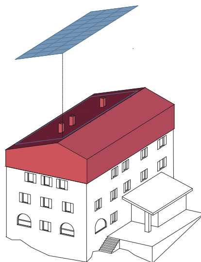
PROGETTO: Falda asimmetrica per garantire una maggiore superficie per l'installazione del fotovoltaico
